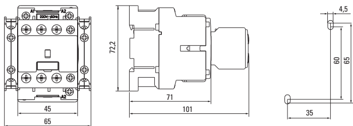
Рис. 3 – Габаритные и установочные размеры контакторов KM3 9A, KM3 12A, KM3 18A, KM3 22A
