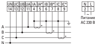
Рисунок 5 – Схема подключения прибора DMC
