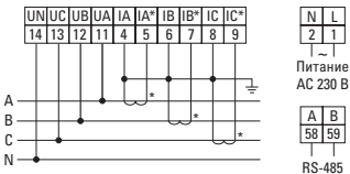
Рисунок 6 – Схема подключения прибора DMC-g
