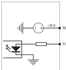
Рис. 7 - Дискретный вход
