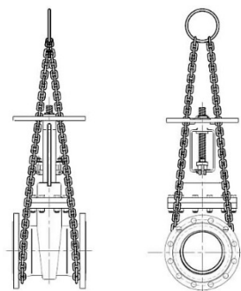
Правильная строповка задвижки
