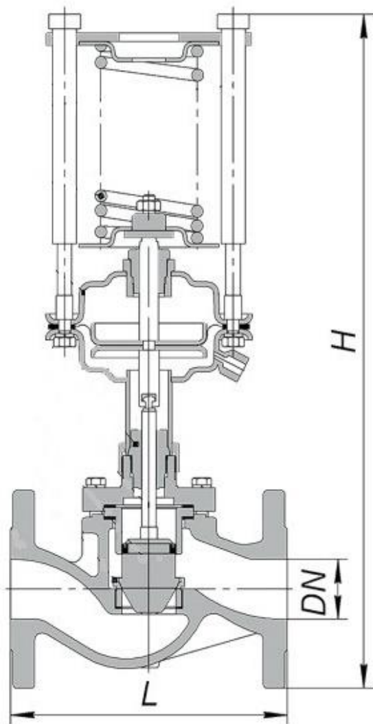
Рисунок 2 - Размеры
