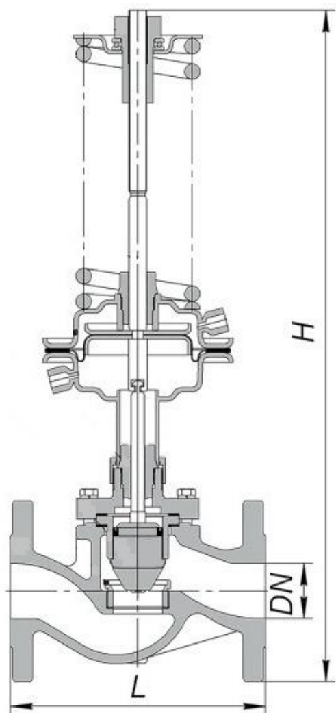
Рисунок 2 - Размеры
