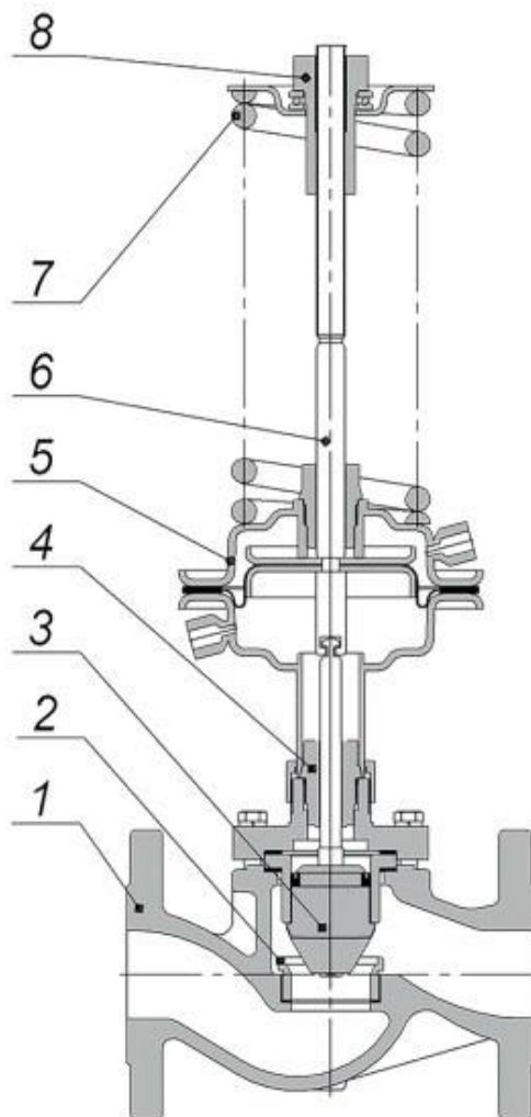
Рисунок 1 - Детализовка
