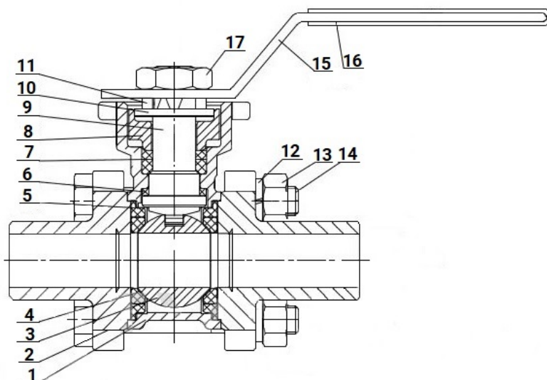
Рисунок 2 - Деталировка
