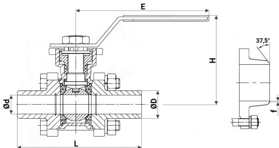
Рисунок 3 – Размеры
