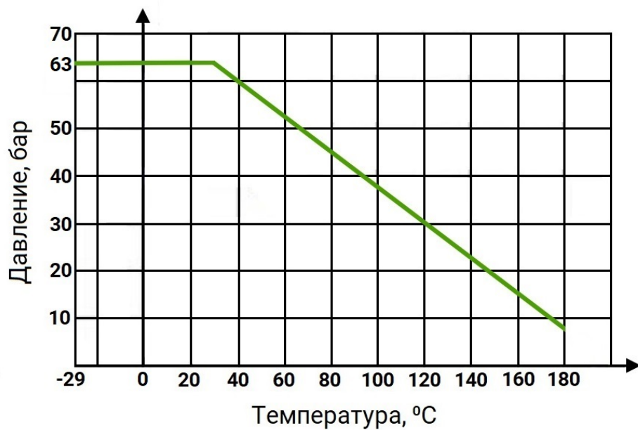
Рисунок 1 – Диаграмма «Температура-давление»
