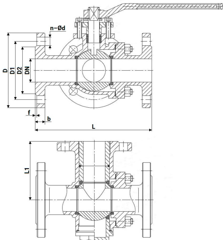
Рисунок 4 – Размеры
