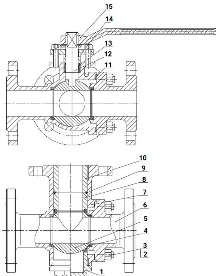
Рисунок 3 – Деталировка
