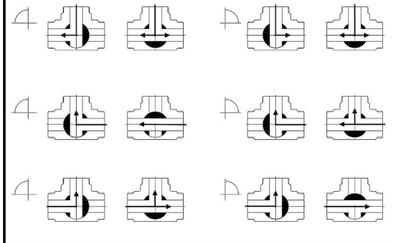
Рисунок 1 – Схемы потока
