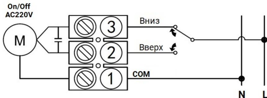
Рисунок 8 – Схема подключения
