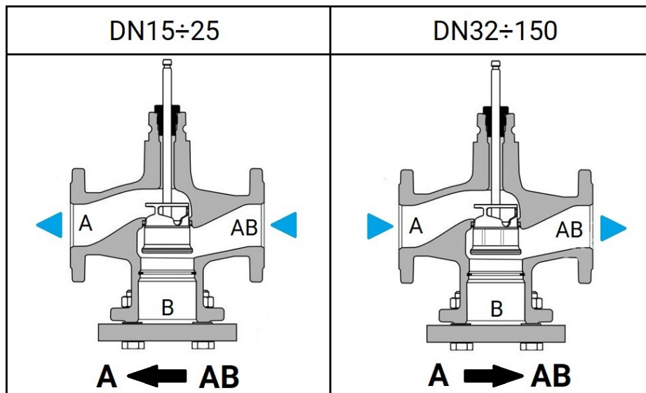
Рисунок 2 – Схемы потока
