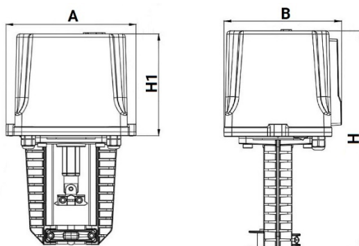
Рисунок 6 – Размеры электроприводов ХСК220-2500 и ХСК220-3000
