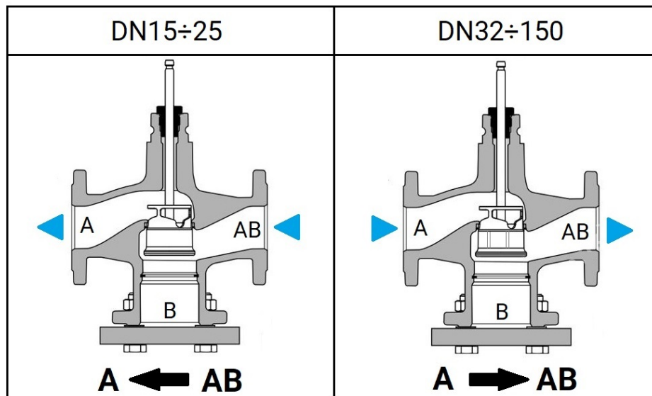
Рисунок 1 – Схемы потока
