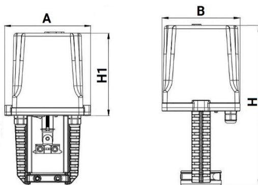
Рисунок 5 – Размеры электропривода ХСК220-1500
