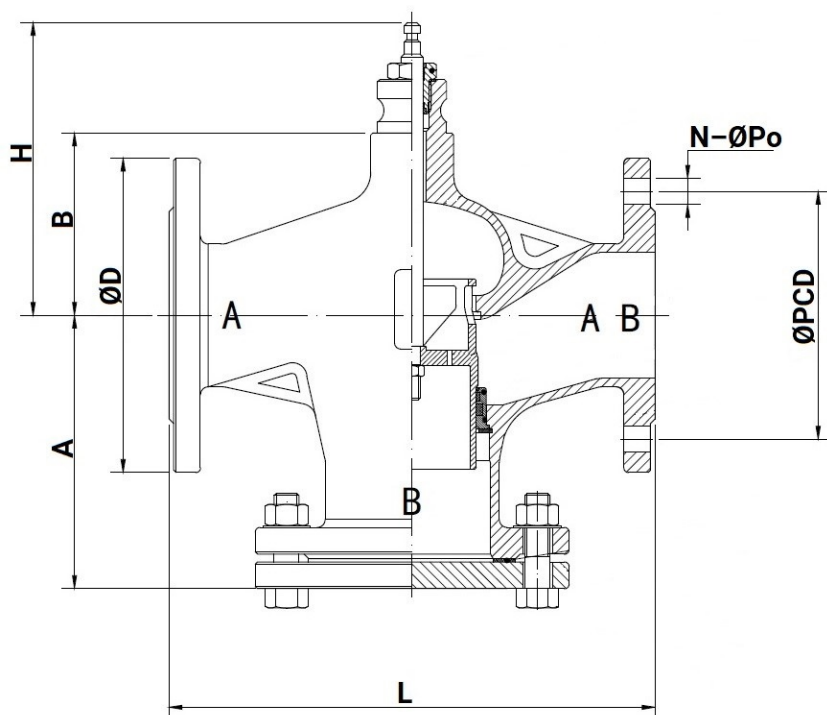
Рисунок 4 – Размеры корпуса клапана DN80÷150
