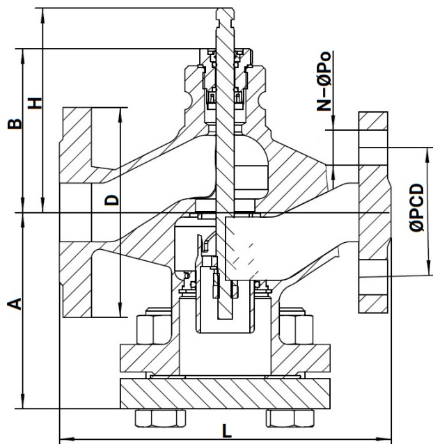
Рисунок 3 – Размеры корпуса клапана DN15÷65
