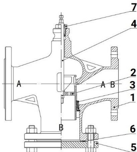
Рисунок 2 – Основные детали
