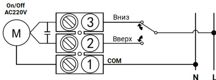
Рисунок 7 – Схема подключения
