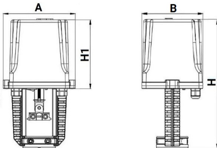
Рисунок 6 – Размеры электропривода ХСК220-1500
