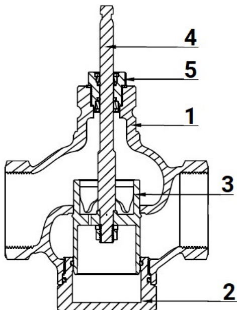
Рисунок 4 – Основные детали корпуса клапана DN32÷50
