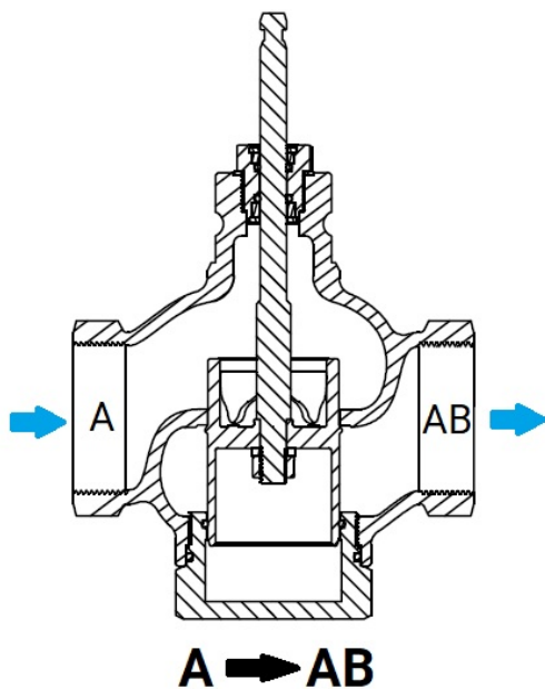
Рисунок 2 – Схема потока
