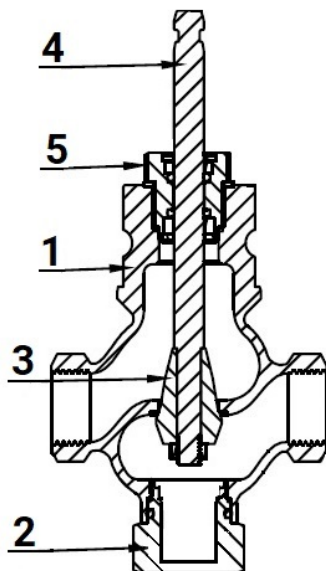
Рисунок 3 – Основные детали корпуса клапана DN15÷25
