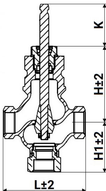
Рисунок 4 – Размеры
