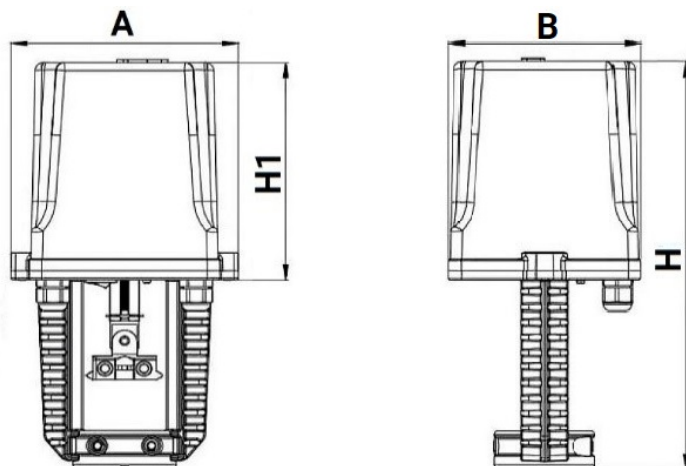
Рисунок 5 – Размеры электропривода ХСК220-1500
