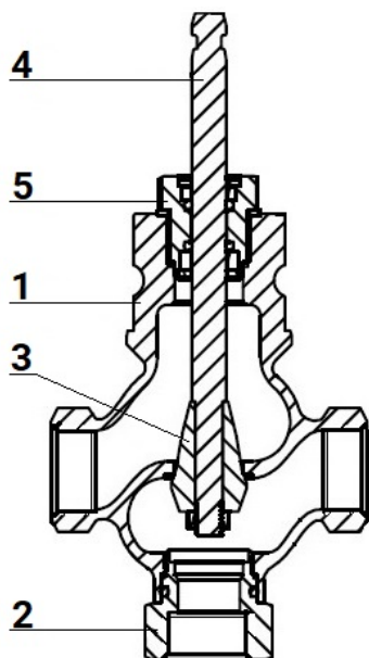
Рисунок 3 – Основные детали
