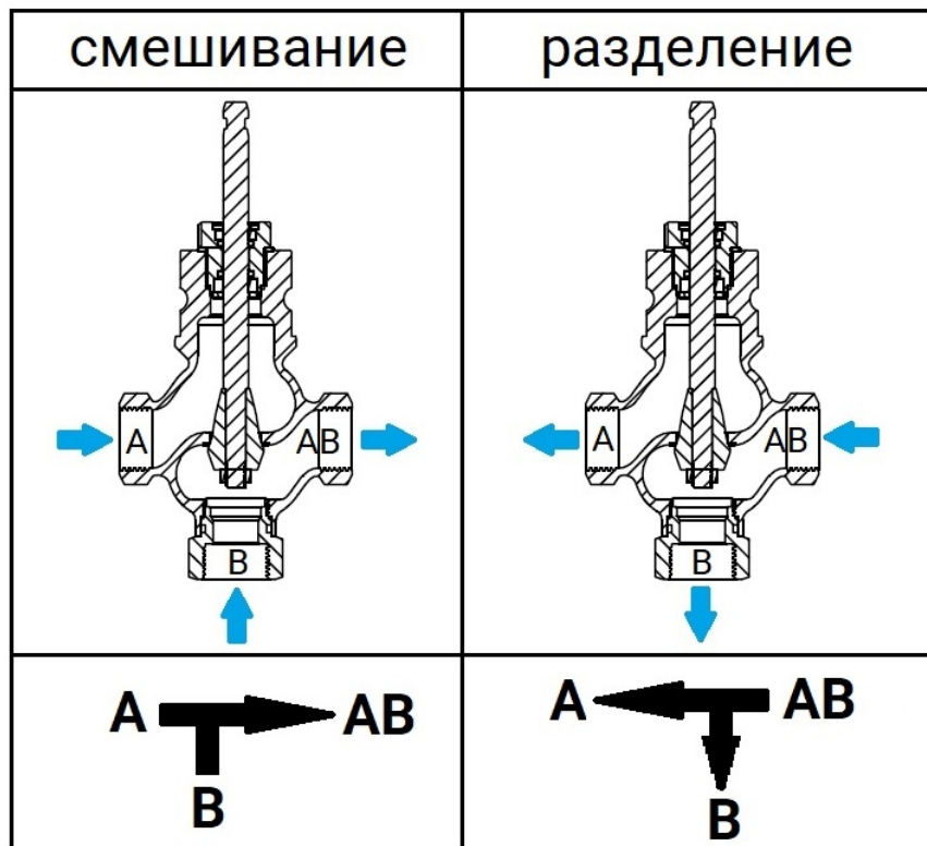
Рисунок 2 – Схемы потока
