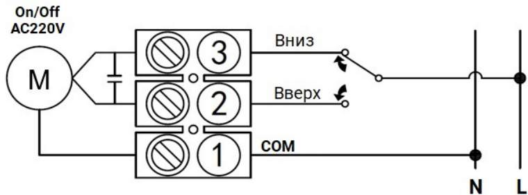
Рисунок 6 – Схема подключения
