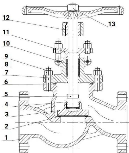
Рисунок 1 - Детализовка
