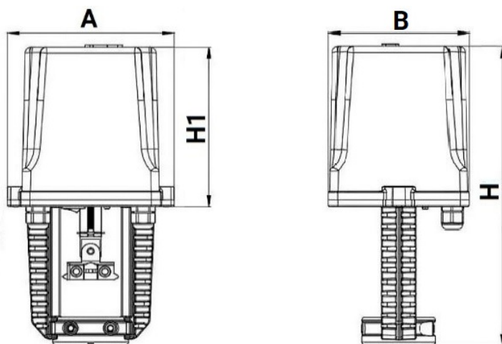
Рисунок 5 – Размеры электропривода ХСК220-1500
