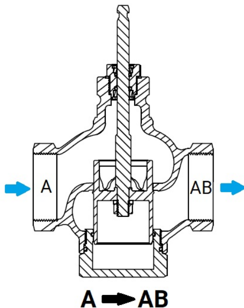
Рисунок 1 – Схема потока
