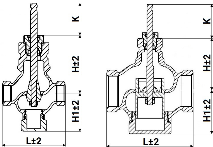
Рисунок 4 – Размеры
