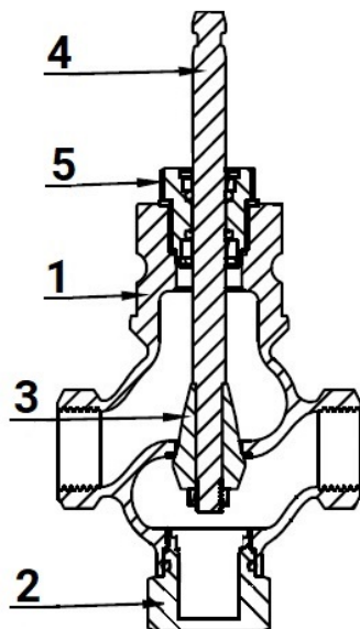
Рисунок 2 – Основные детали корпуса клапана DN15÷25
