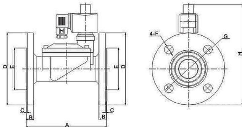
Рисунок 2 – Размеры клапана (материал корпуса - чугун)
