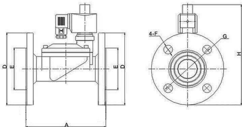
Рисунок 1 – Размеры клапана (материал корпуса - нержавеющая сталь AISI 304)
