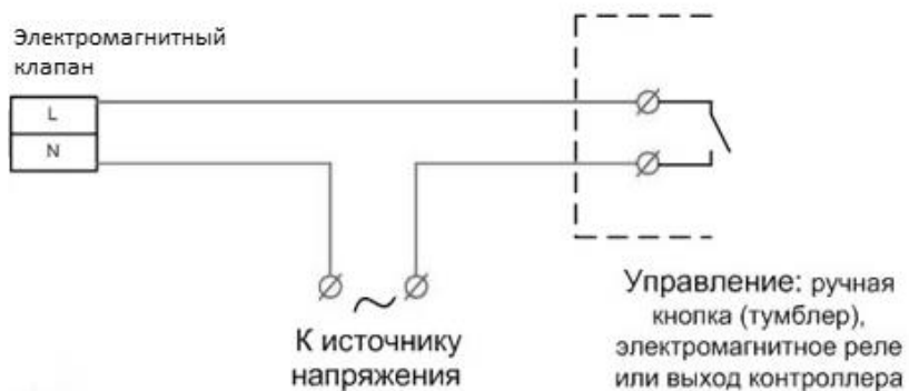
Схема подключения
