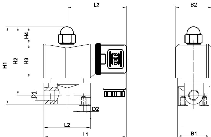
Рисунок 2 – Размеры клапанов Дуг-8 корпус латунь
