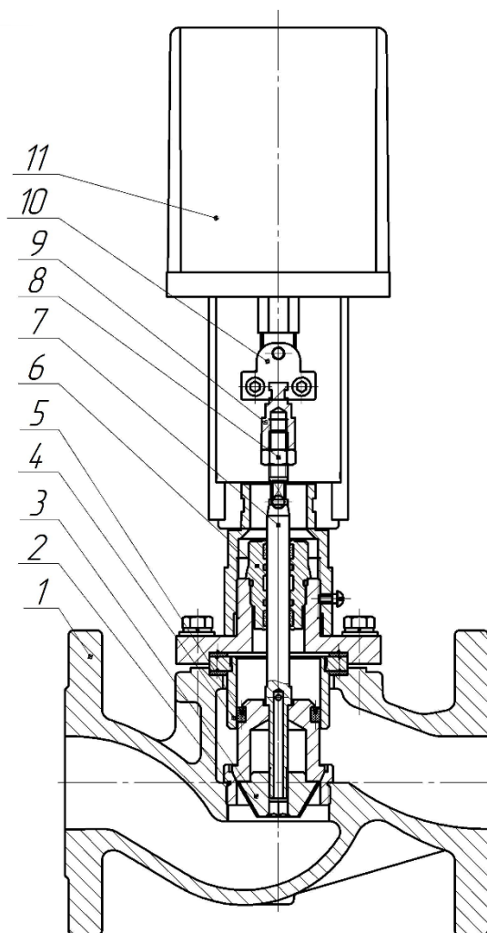
Рисунок 1 - Деталировка
