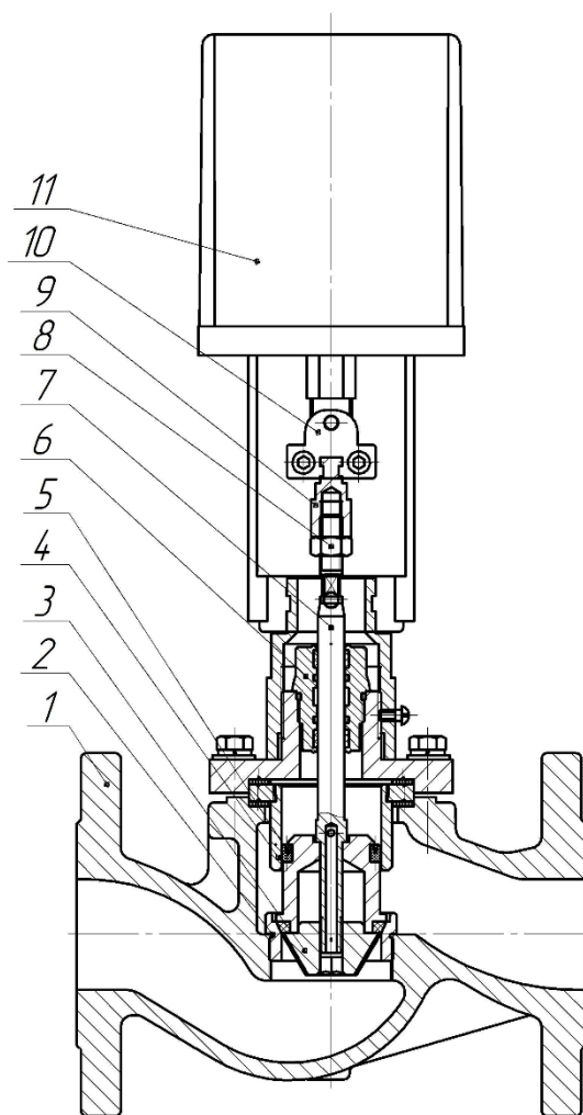
Рисунок 1 - Деталировка
