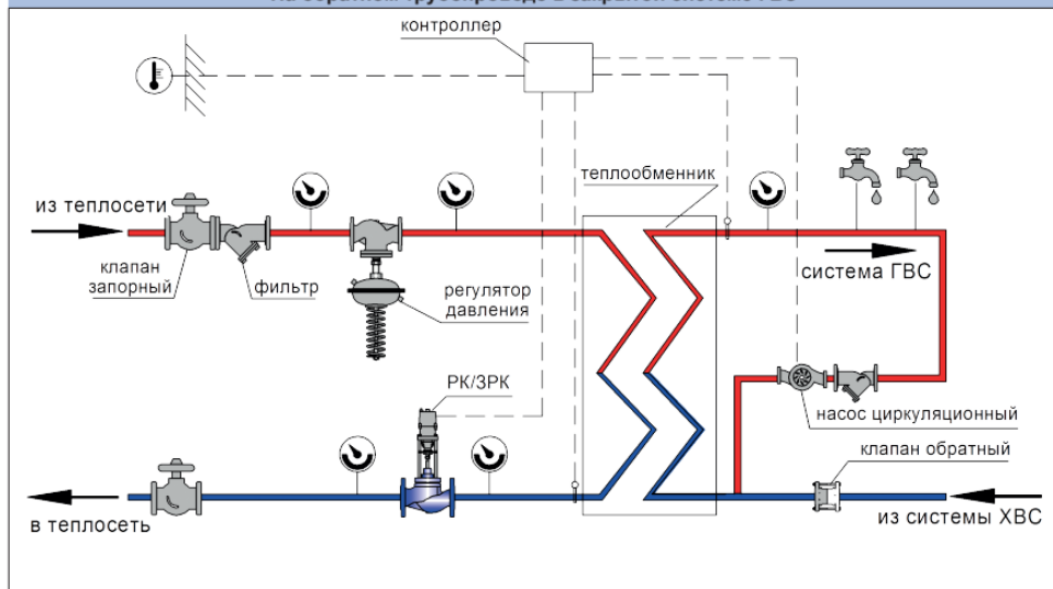
Рисунок 4 - Схемы подключения РК
