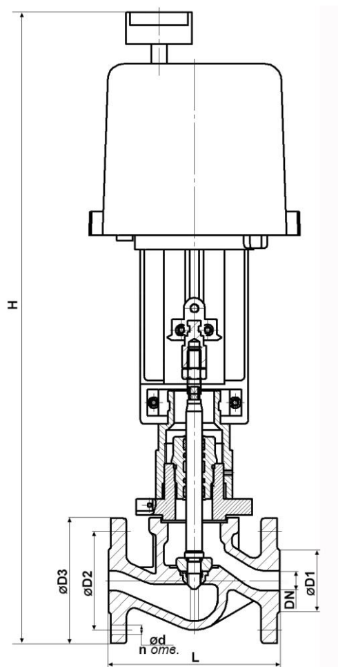
Рисунок 2 - Размеры
