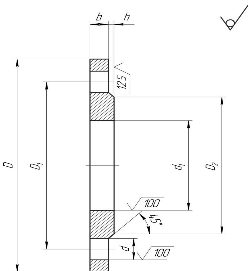
Рисунок 1 - Размеры
