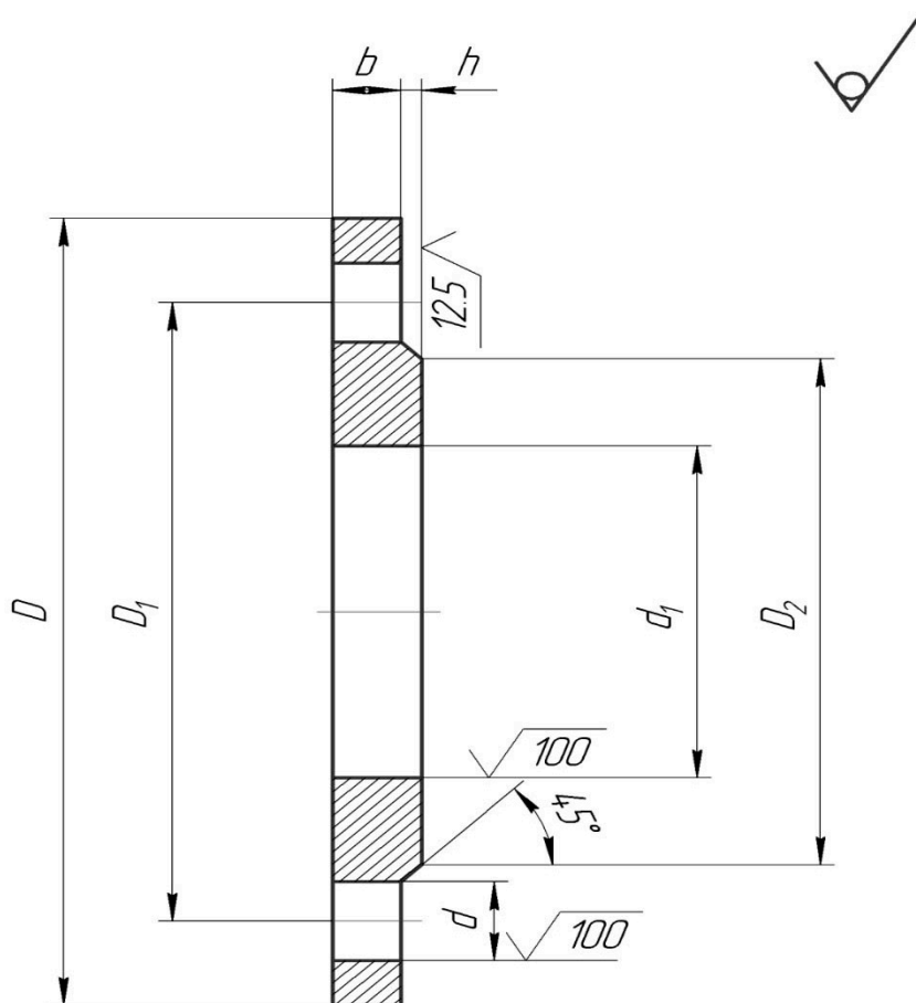
Рисунок 1 - Размеры
