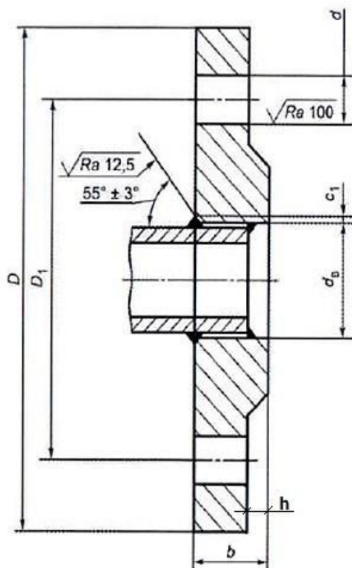
Рисунок 1 - Размеры
