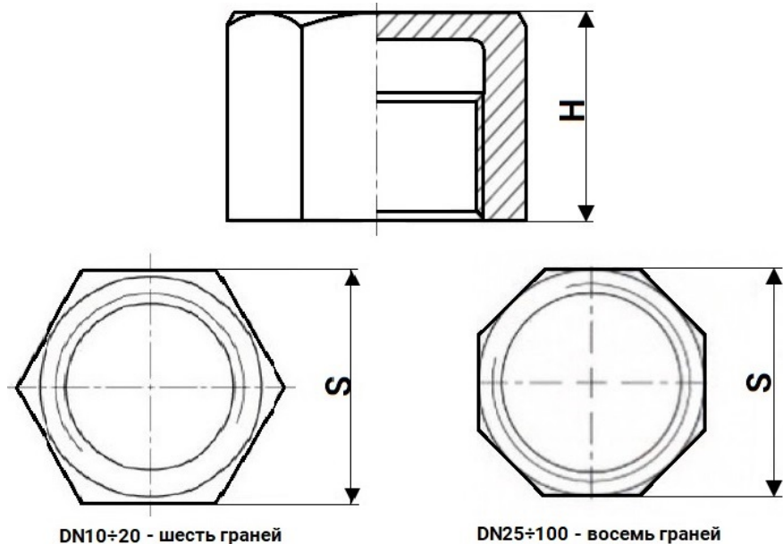
Рисунок 1 – Размеры
