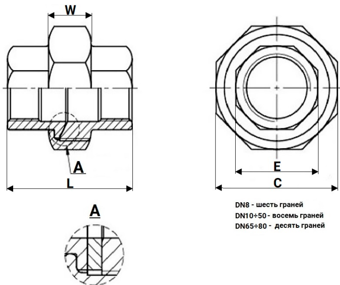
Рисунок 1 – Размеры
