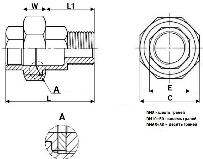
Рисунок 1 – Размеры
