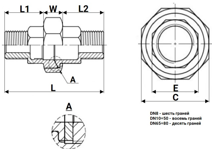
Рисунок 1 – Размеры
