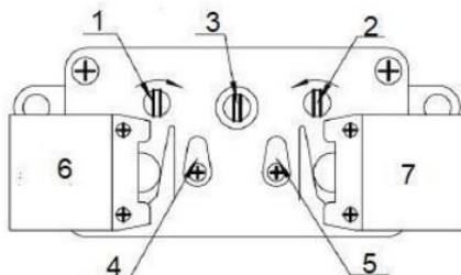
Рисунок 9 – Регулировка хода закрытия
