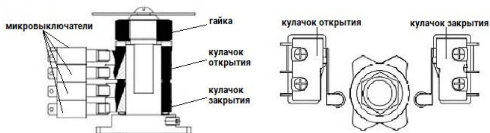
Рисунок 4 – Концевые выключатели
