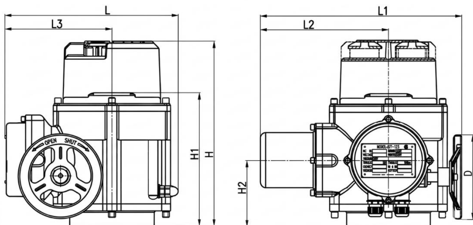
Рисунок 3 – Размеры электропривода
