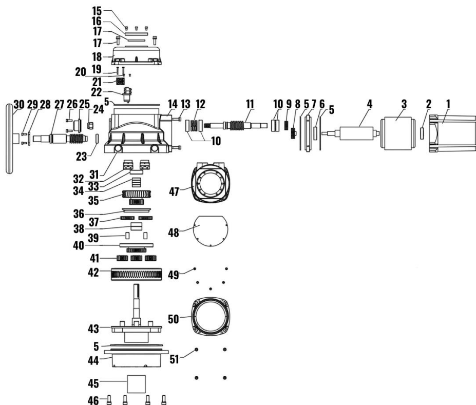
Рисунок 2 – Основные детали
