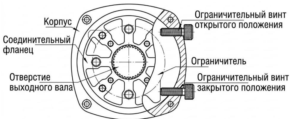
Рисунок 6 – Элементы регулировки
