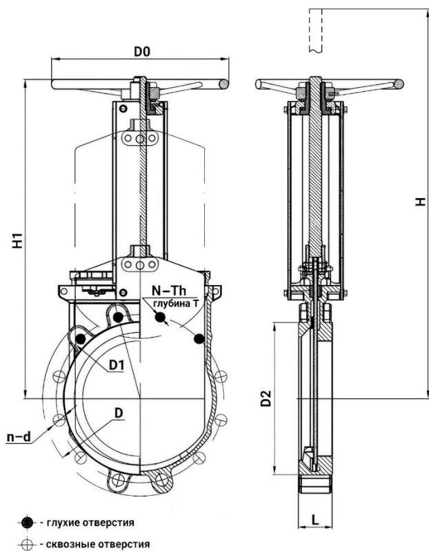
Рисунок 3 – Размеры изделия
