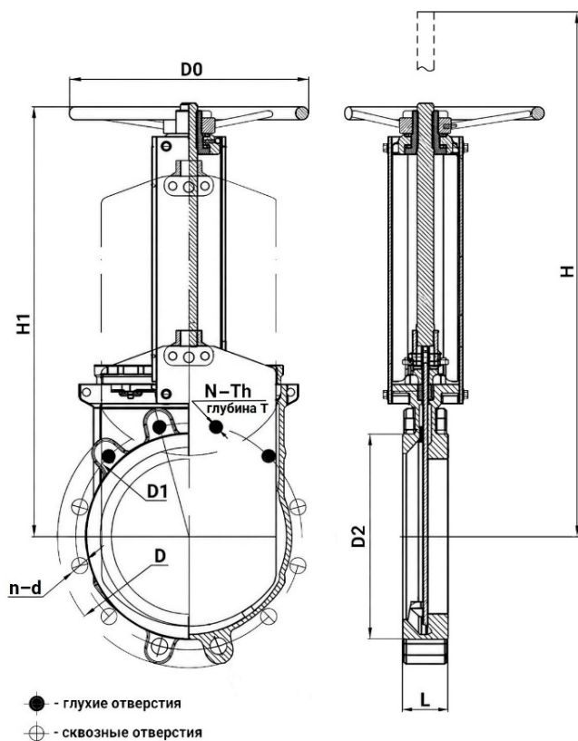
Рисунок – Размеры изделия
