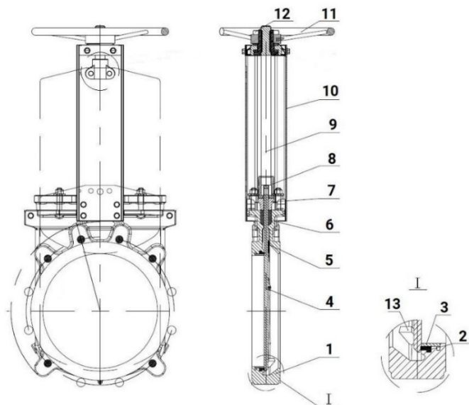
Рисунок 1 – Деталировка
