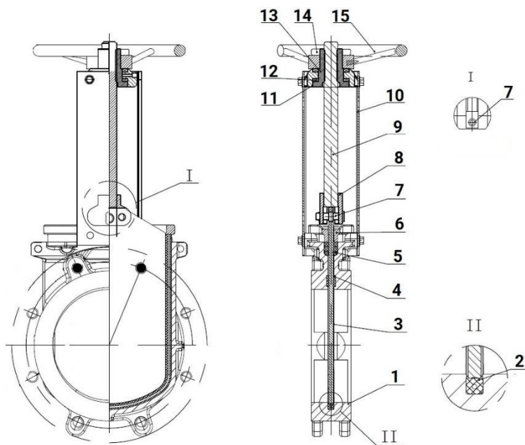
Рисунок 1 – Деталировка
