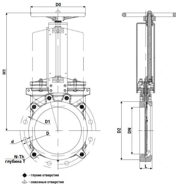
Рисунок 2 – Размеры
