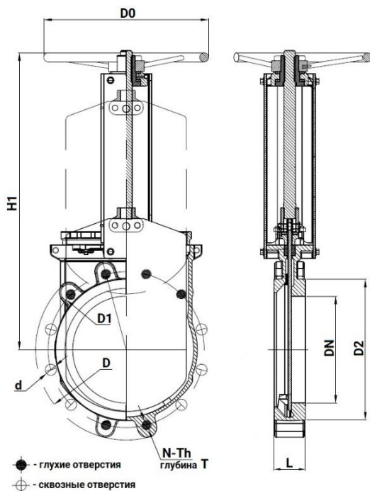
Рисунок 2 – Размеры
