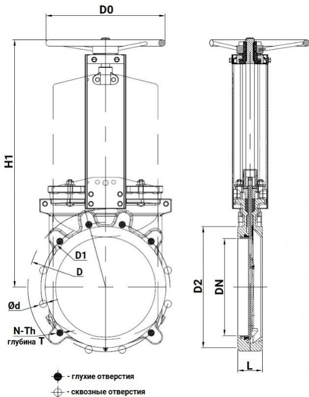
Рисунок 2 – Размеры
