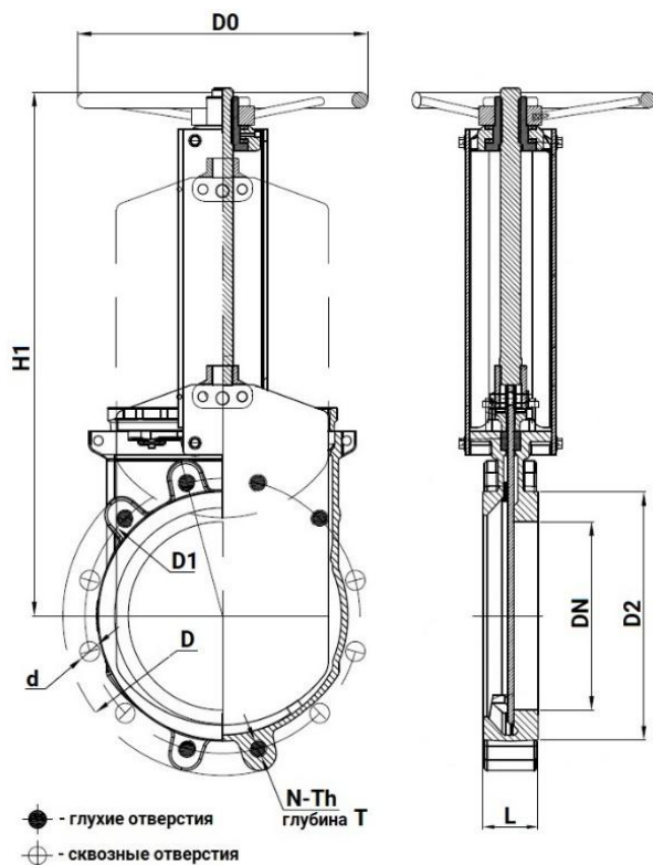
Рисунок 2 – Размеры
