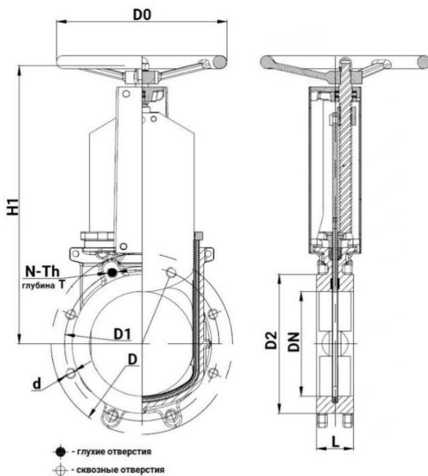
Рисунок 2 – Размеры
