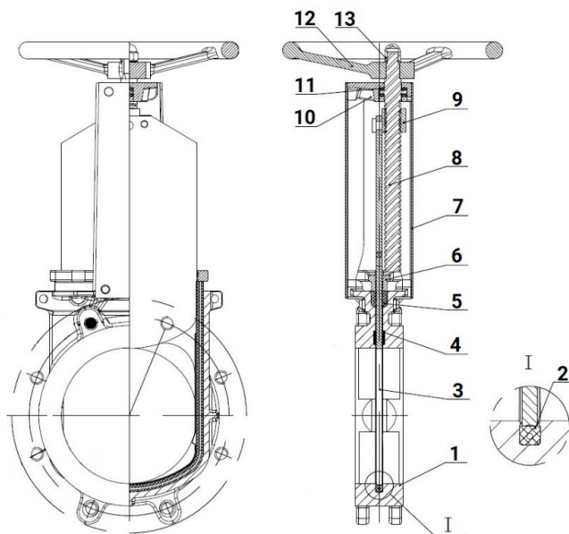
Рисунок 1 – Деталировка
