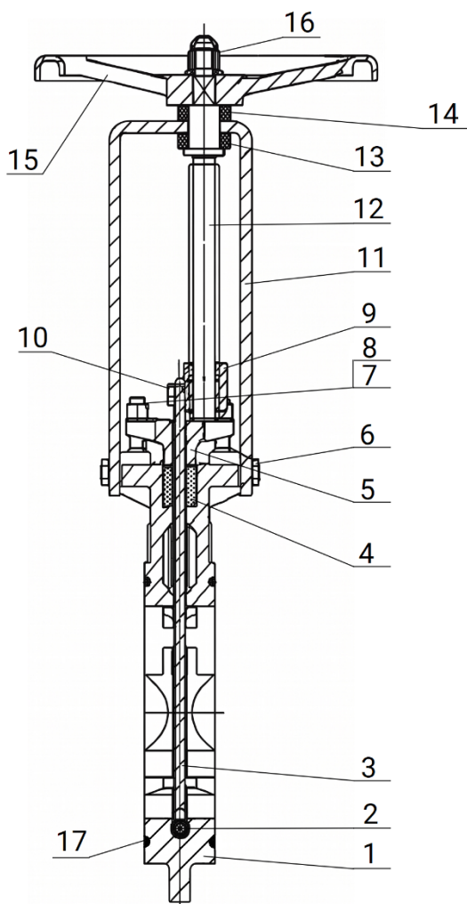
Рисунок 2 – Составные части изделия
