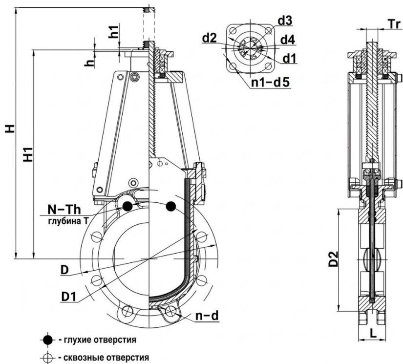
Рисунок 3 – Размеры изделия
