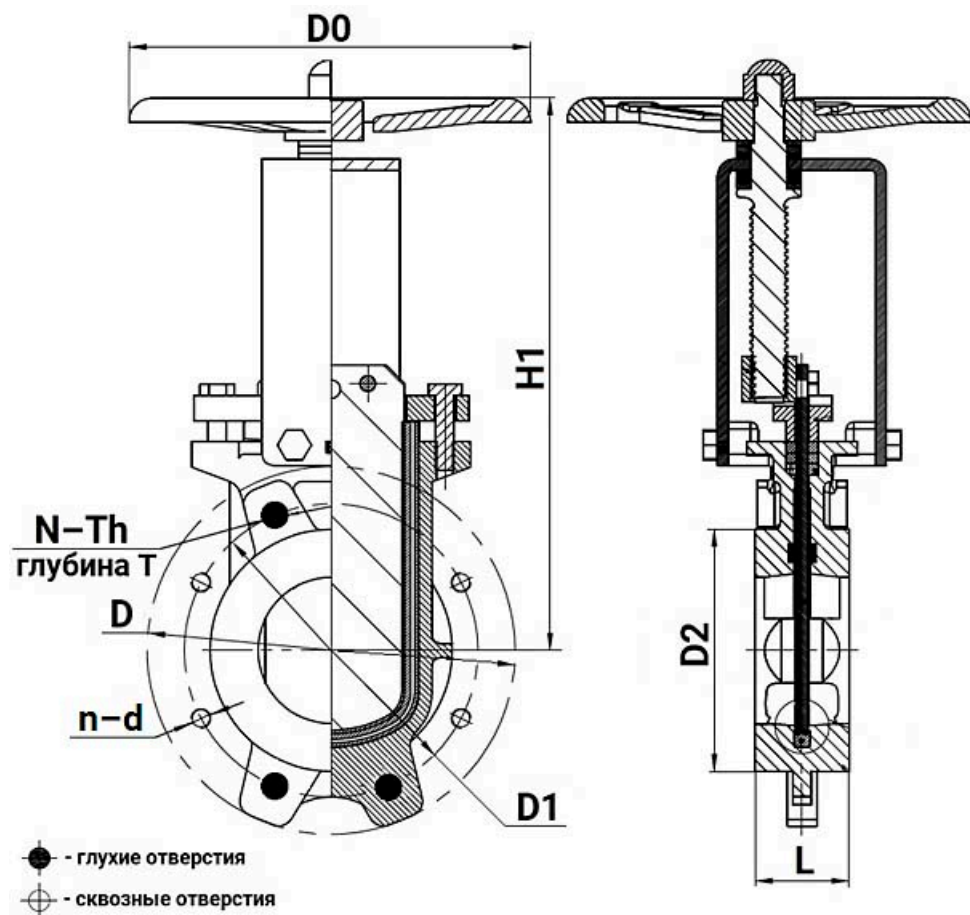
Рисунок 3 – Размеры изделия
