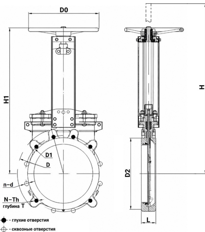
Рисунок 3 – Размеры изделия
