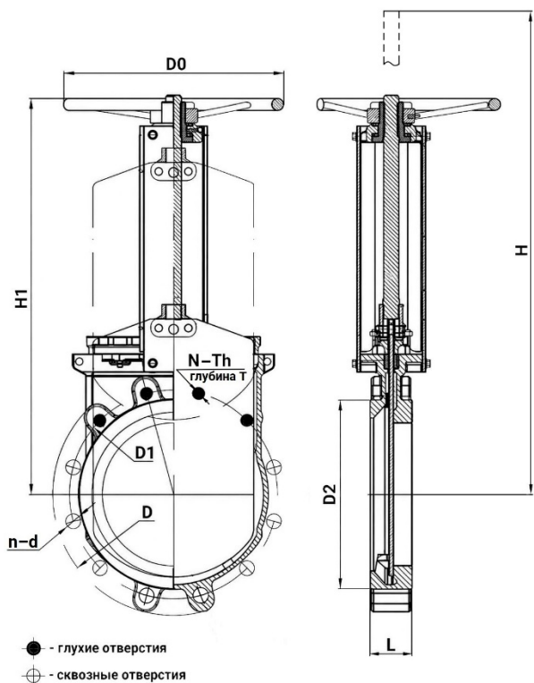
Рисунок 3 – Размеры изделия
