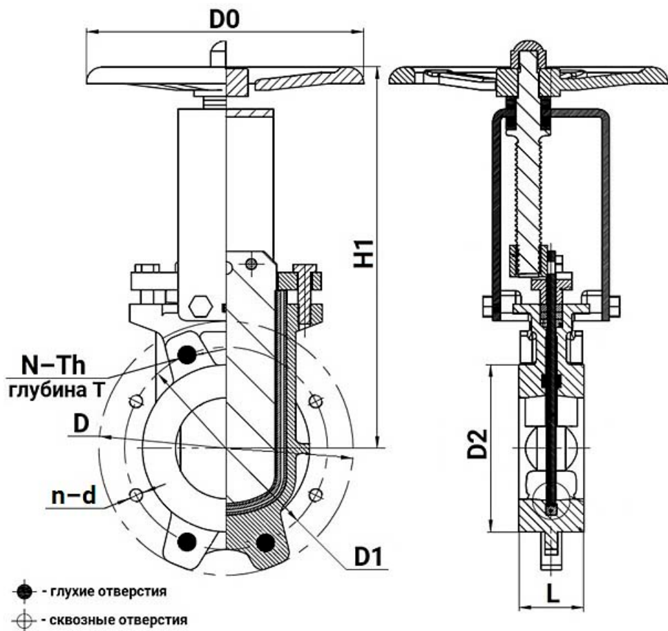
Рисунок 3 – Размеры изделия
