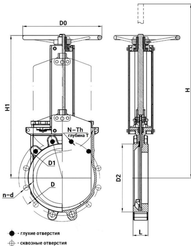
Рисунок 3 – Размеры изделия
