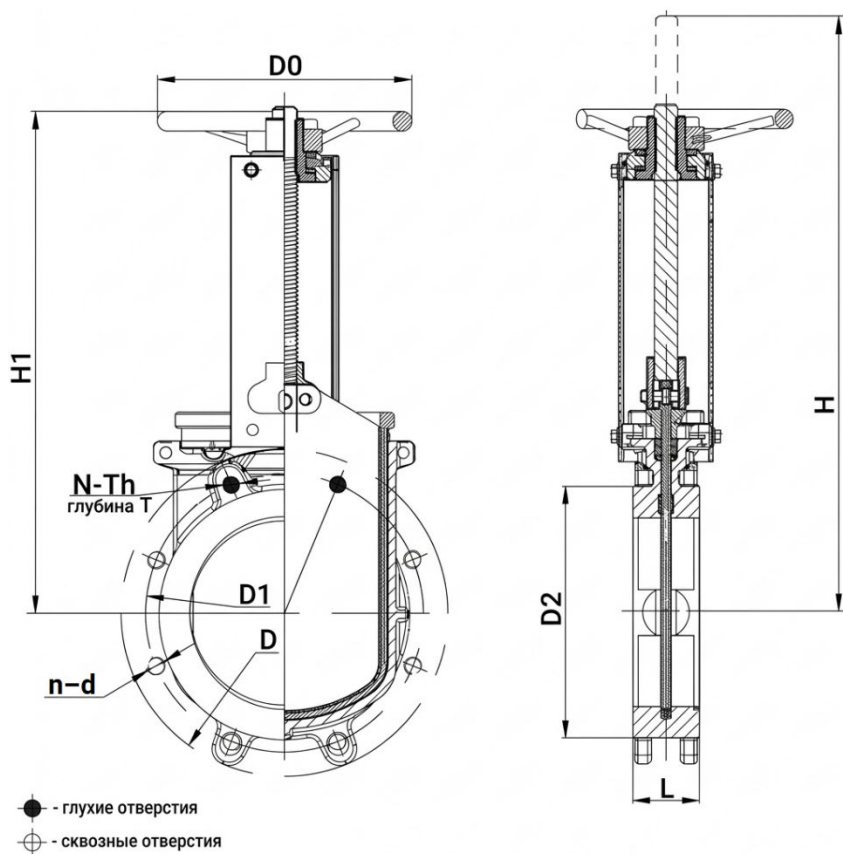
Рисунок 3 – Размеры изделия
