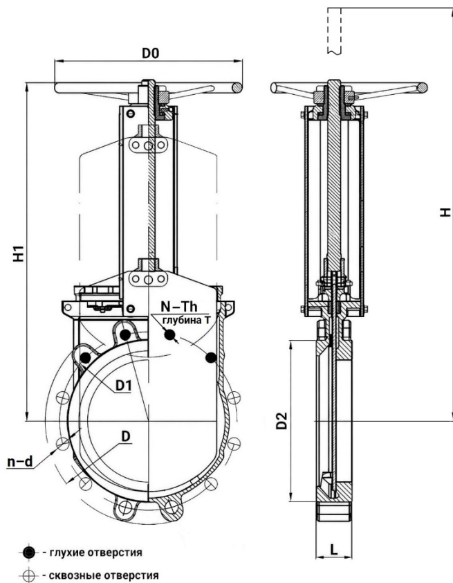
Рисунок 3 – Размеры изделия
