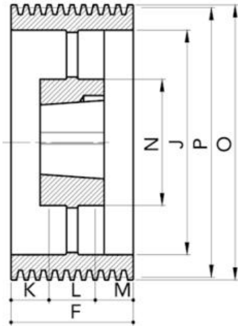
Disegno Tecnico 2D
